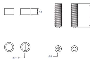
Kit fissaggio singolo con foro passante per porte in vetro Single fixing kit with through hole for glass doors
